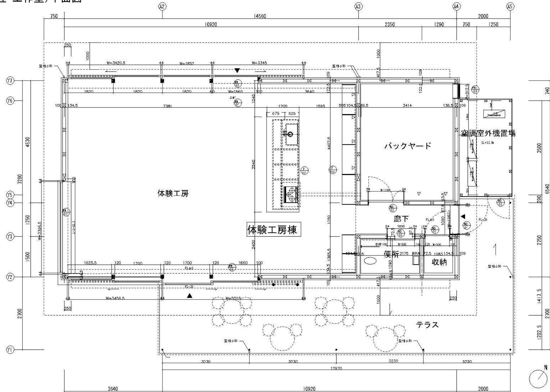
■体験工房（調理・工作室）平面図
