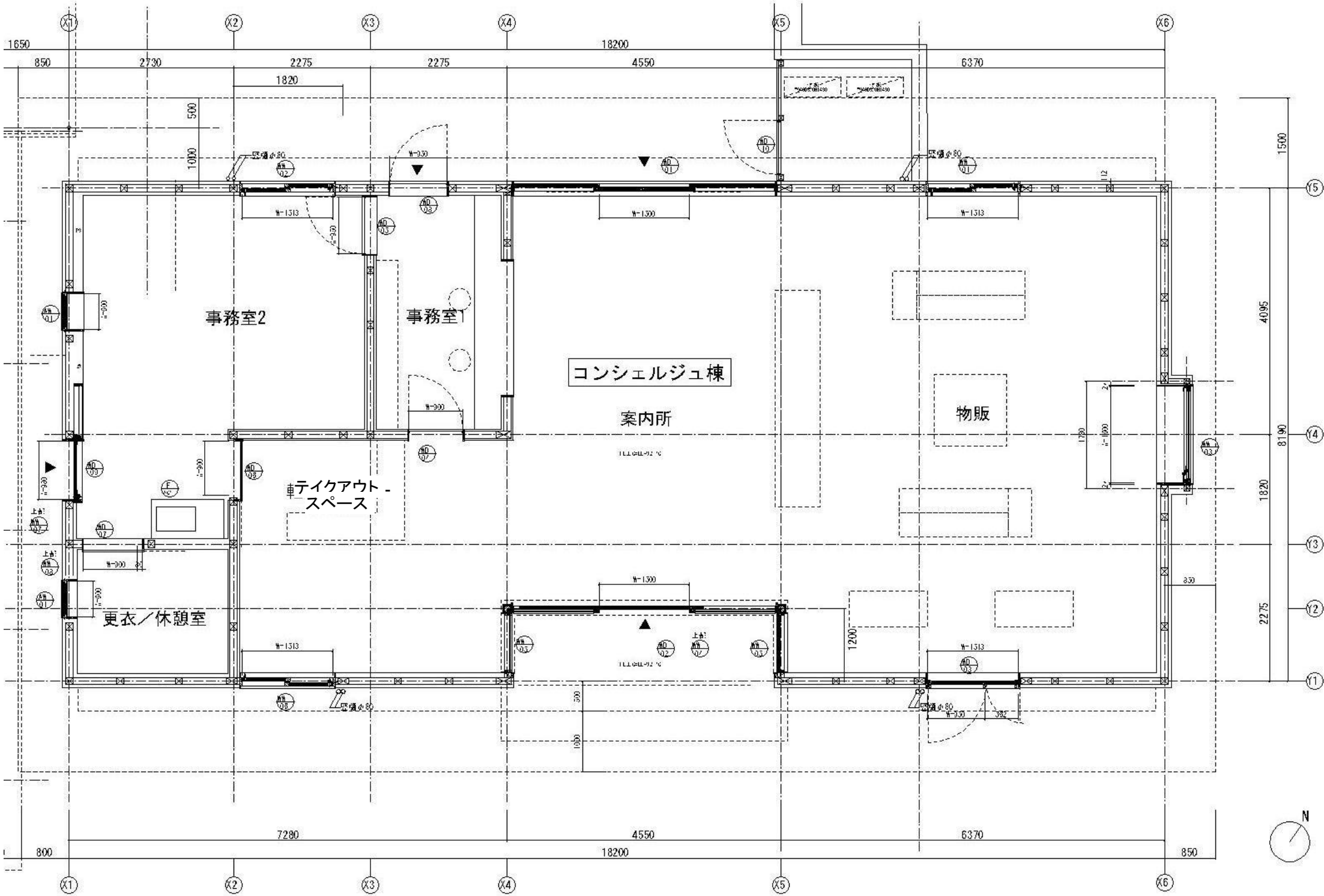
■コンシェルジュ棟平面図
