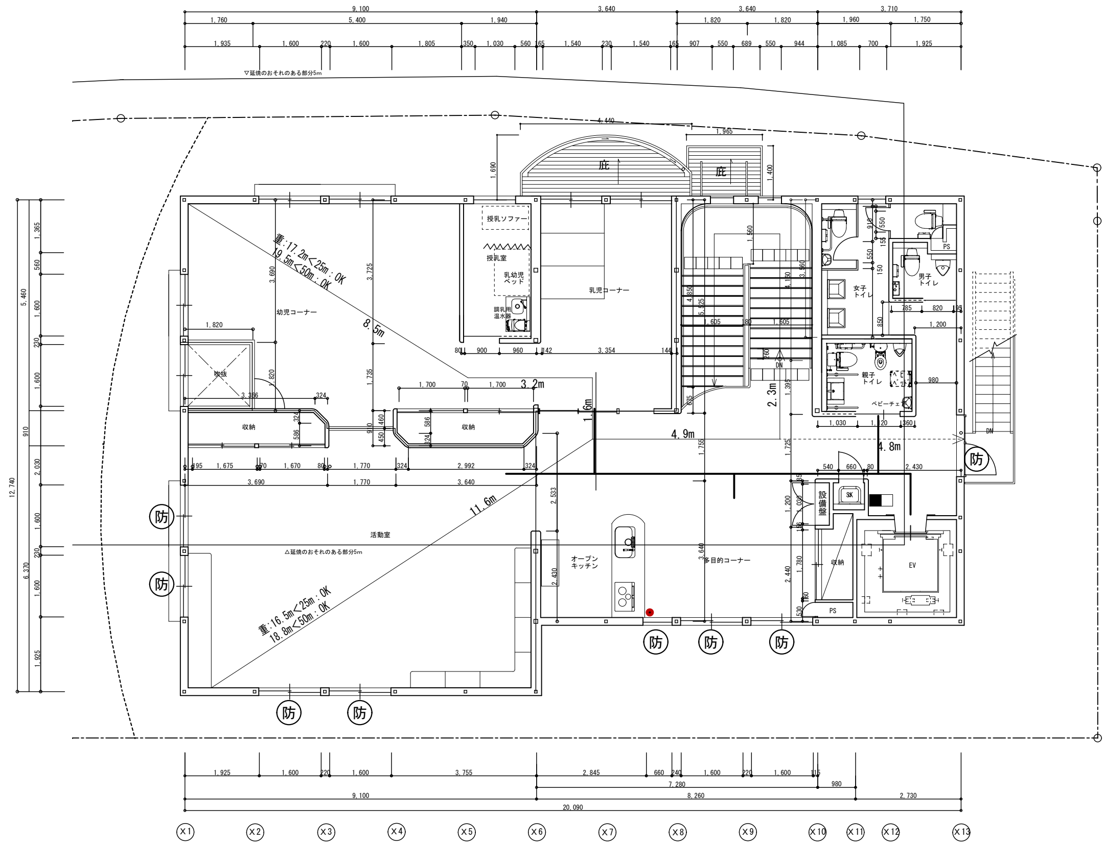
2階平面図
