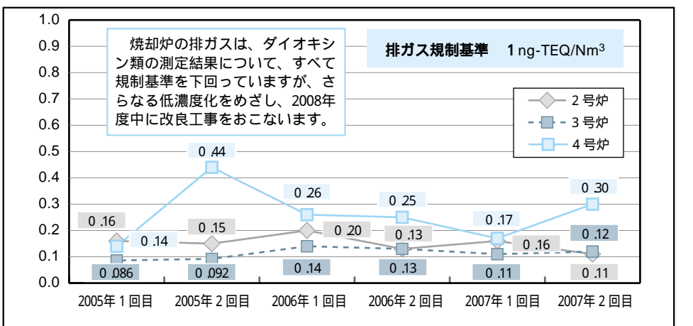
図1. 『焼却炉排ガスの測定結果』(排ガス規制基準値 1ng-TEQ/Nm³)
