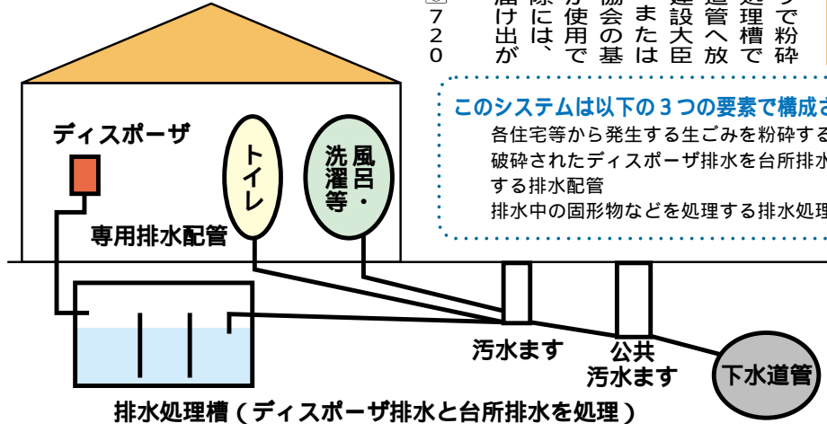
ディスポーザ排水処理システムの概念図
