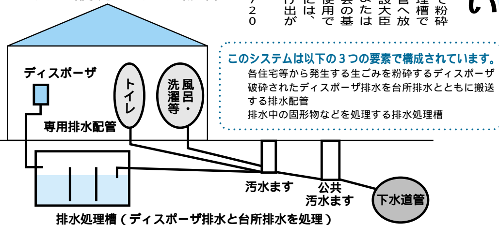
ディスポーザ排水処理システムの概念図
