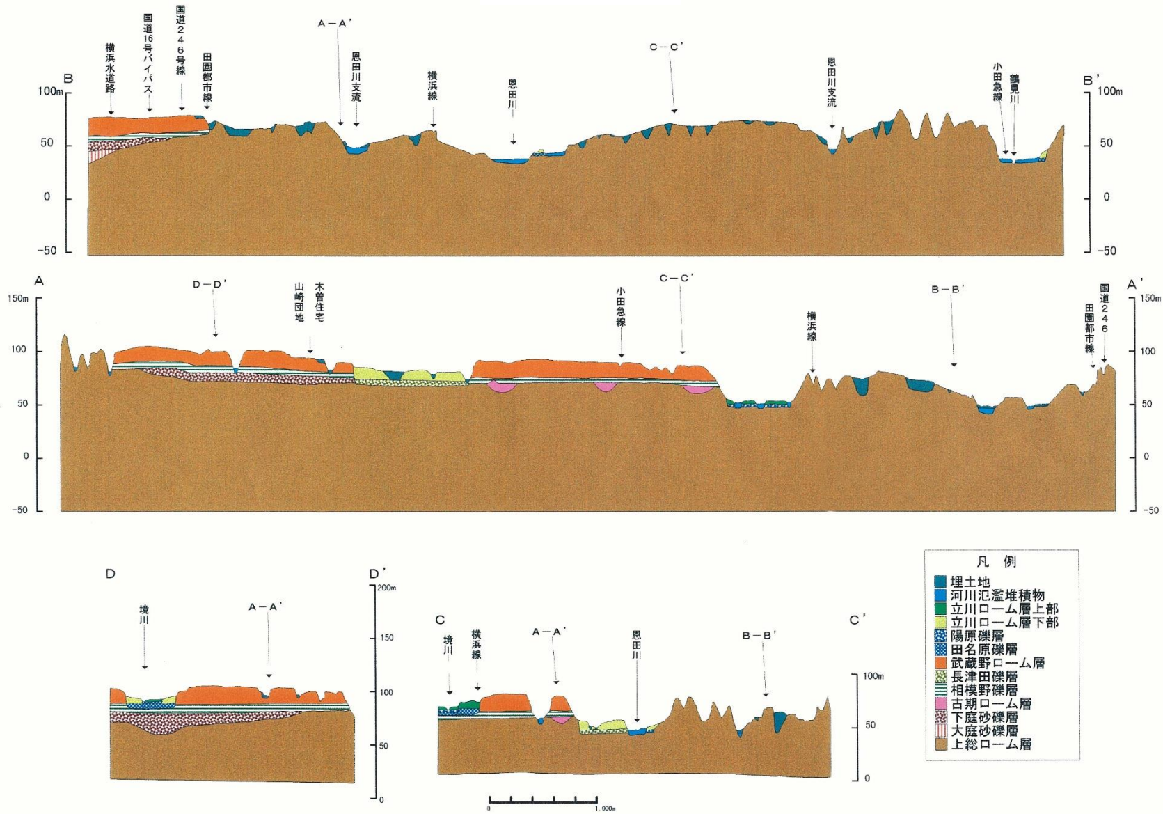
地質断面図
