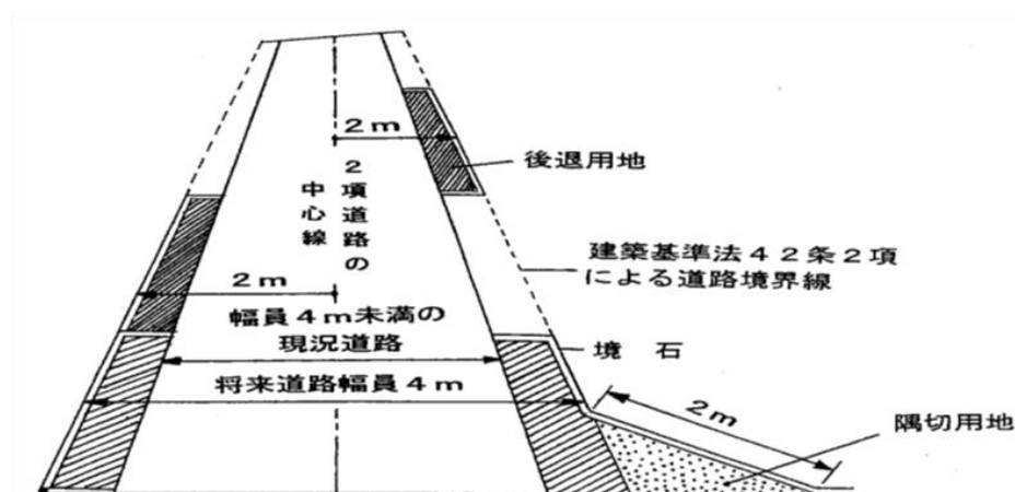
建築基準法第42条第2項道路の後退用地(イメージ)
