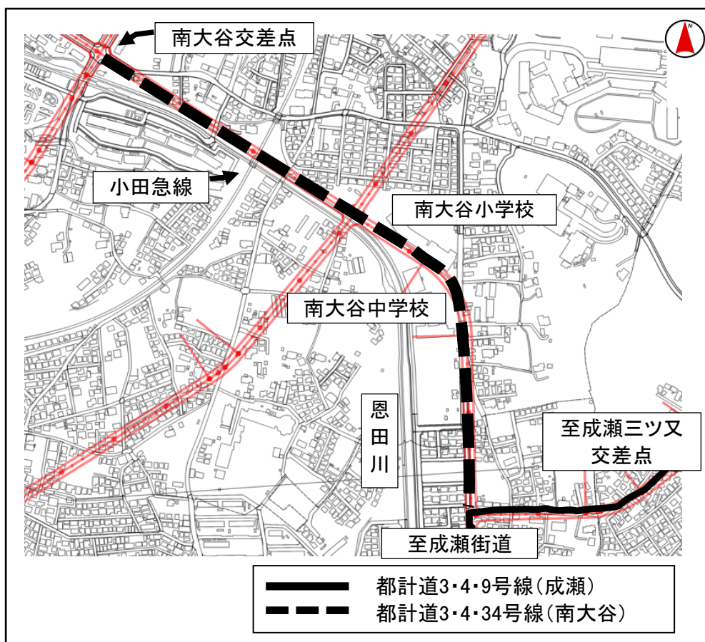
都計道3・4・9(成瀬) 案内図
