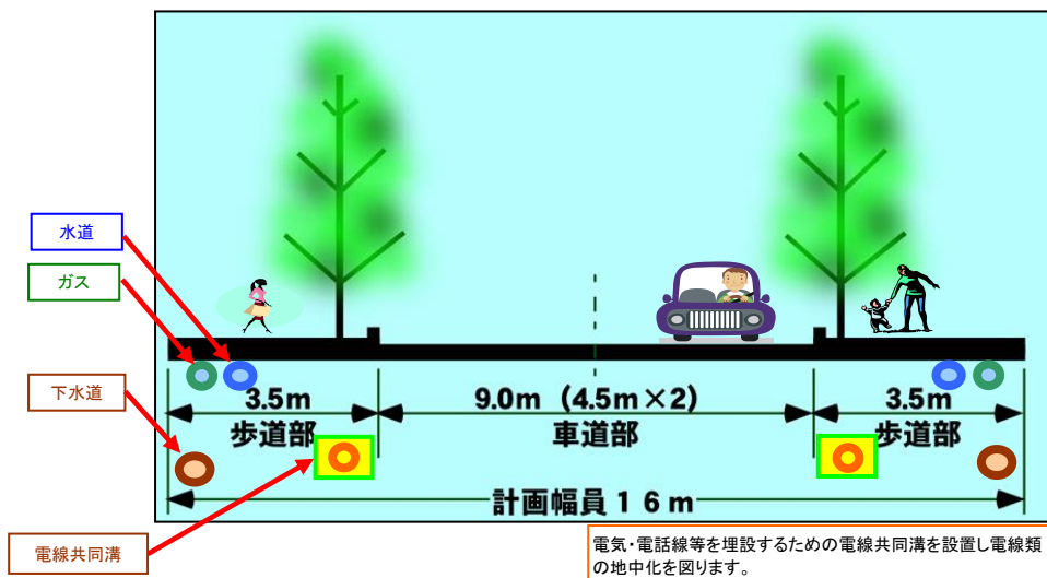
都市計画道路整備(道路幅16mの場合)
