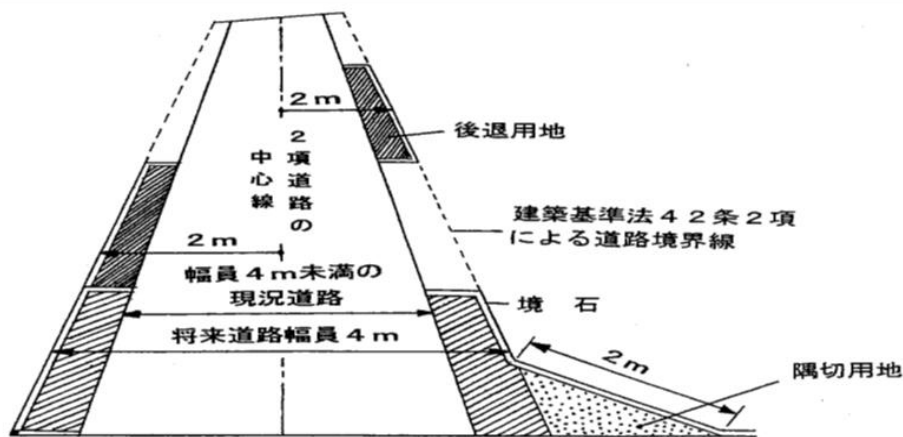
建築基準法第42条第2項道路の後退用地(イメージ)
