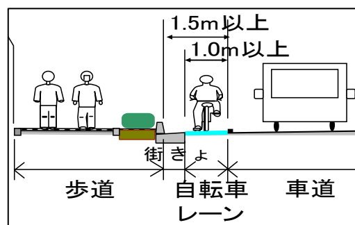
自転車レーンの基本構造
