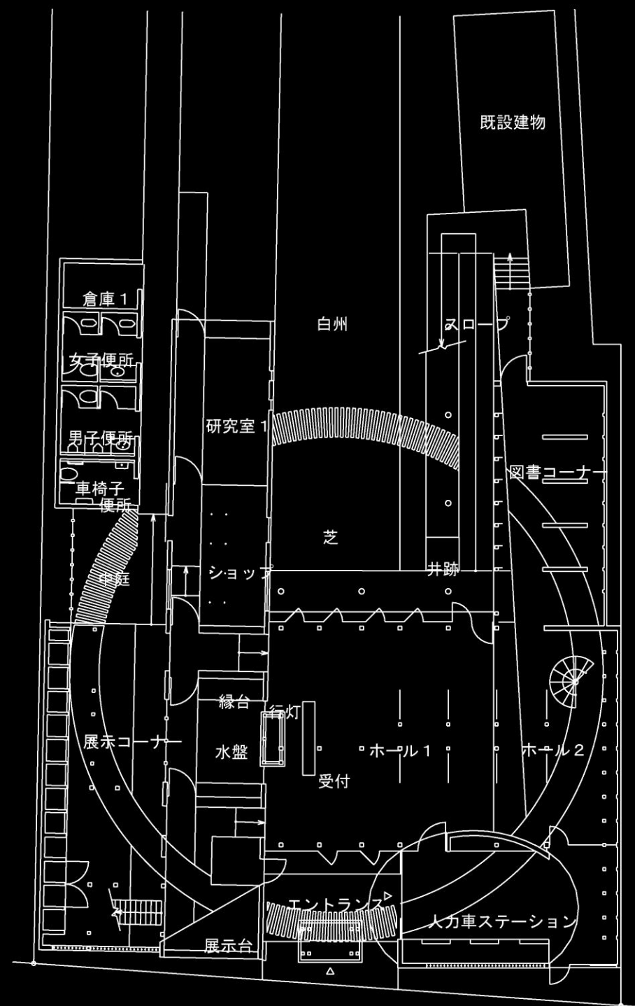
改修後 1階平面図
