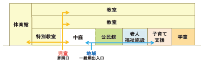
<立面図>
