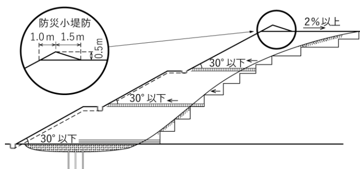
図 4-3 防災小堤
