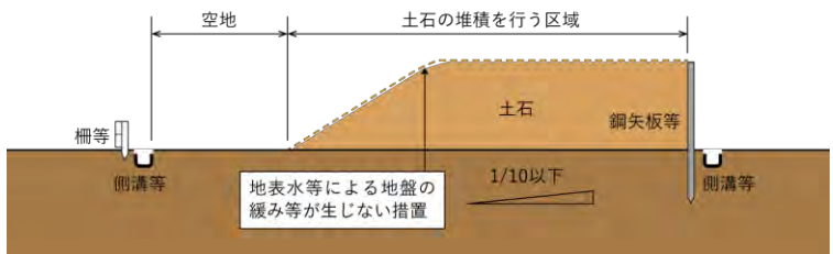
図 3-78 鋼矢板等の設置
