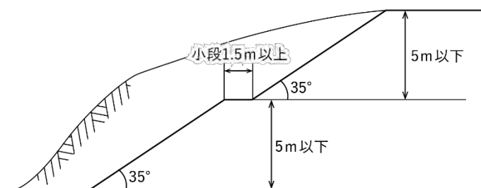
図 3-9 切土法面の形状
