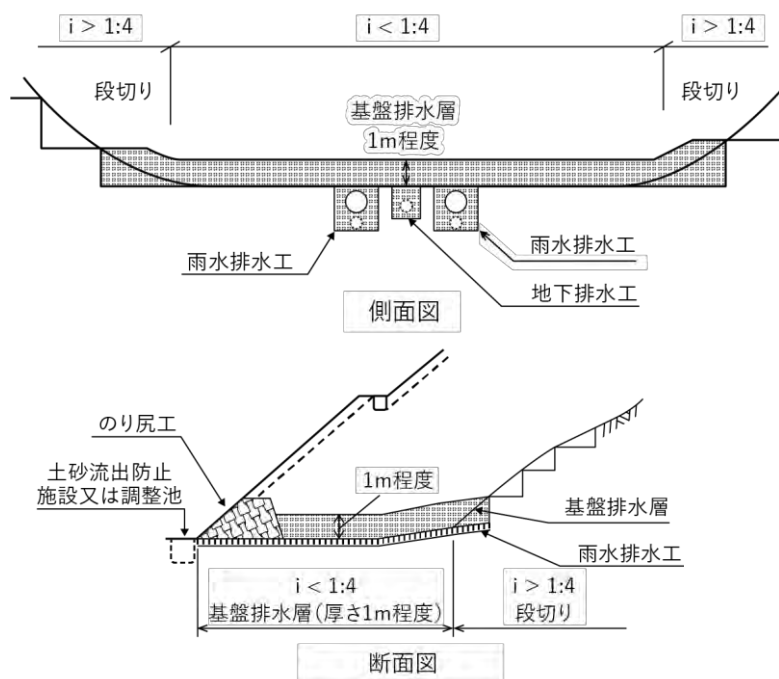
圖 3-70 基盤排水層
