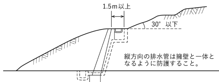
図 3-64 法肩排水工
