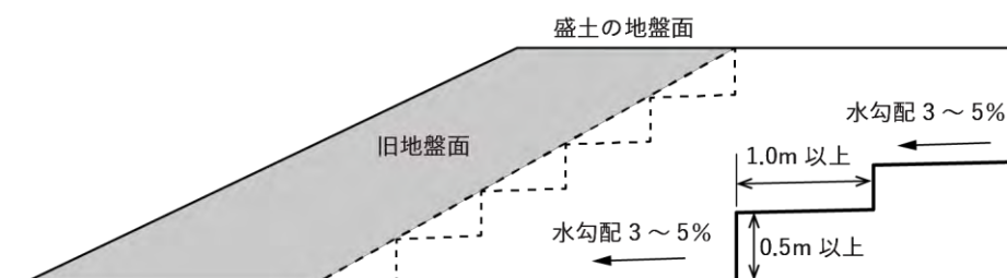
図 3-2 段切りの例
