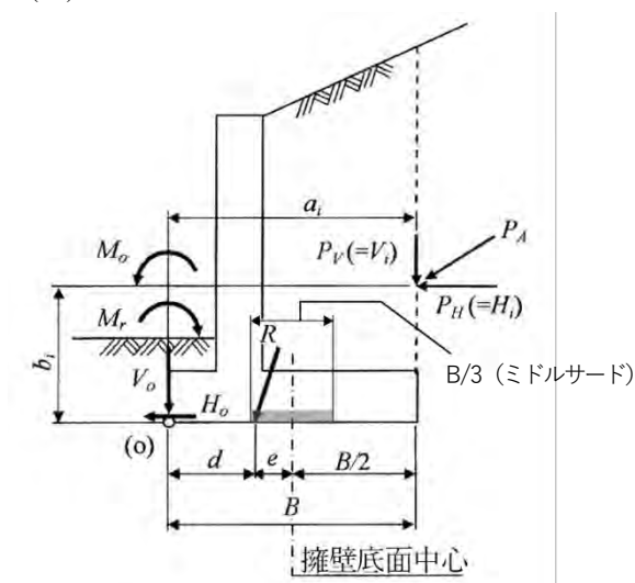
図 3-37 合力作用位置の求め方
