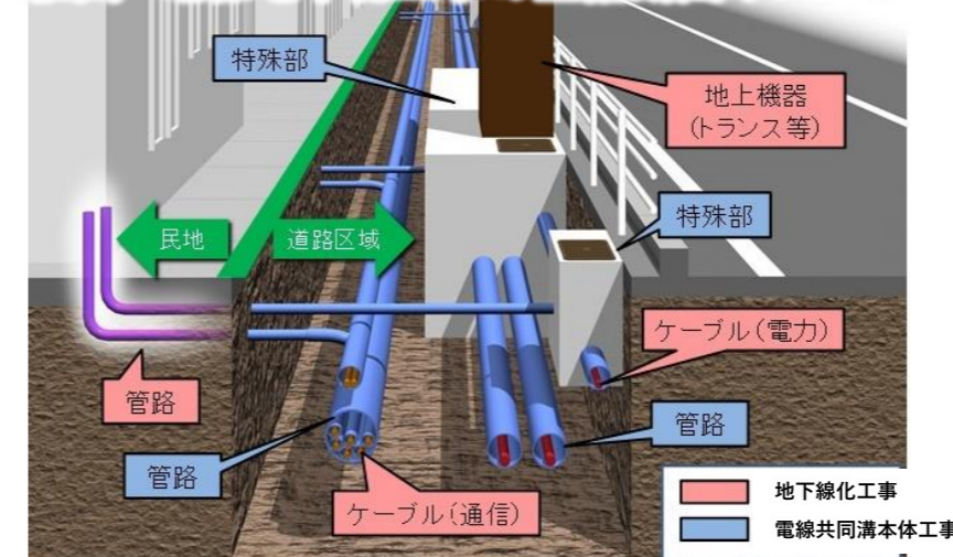
(図1) 電線地中化工事の整備断面イメージ
