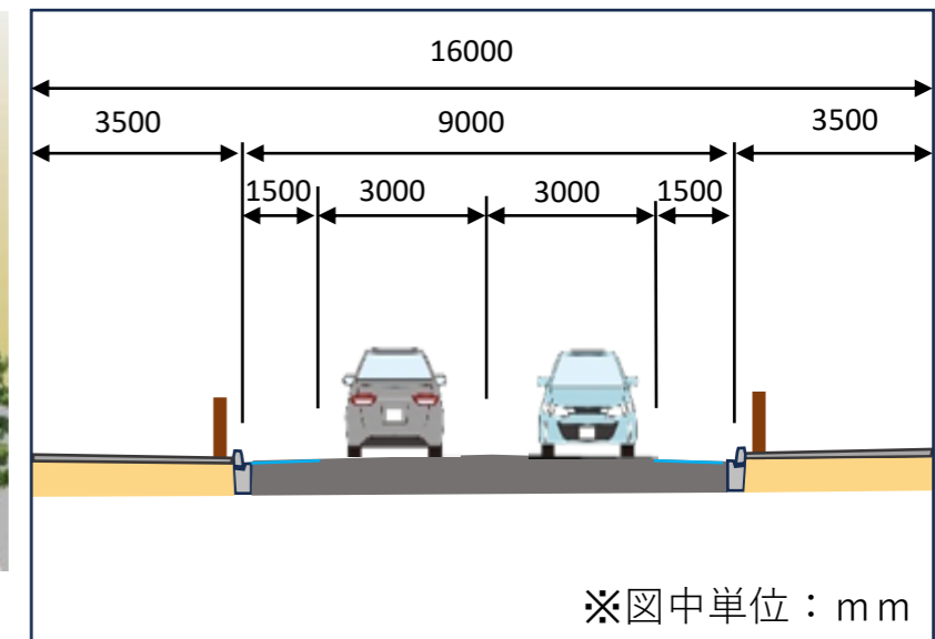
【道路一般部横断面計画図】
