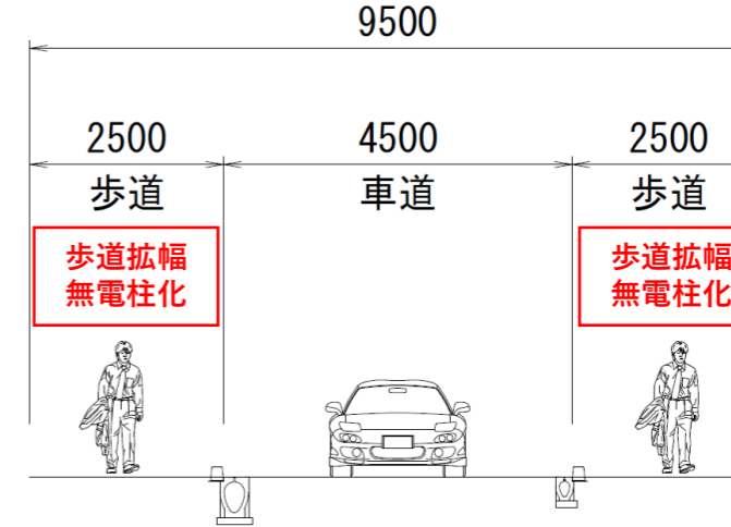
【電線地中化工事の整備断面イメージ】
