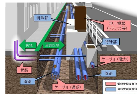
(図2) 地中化の様子
