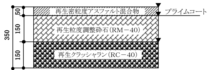
アスファルトコンクリート舗装 35型
