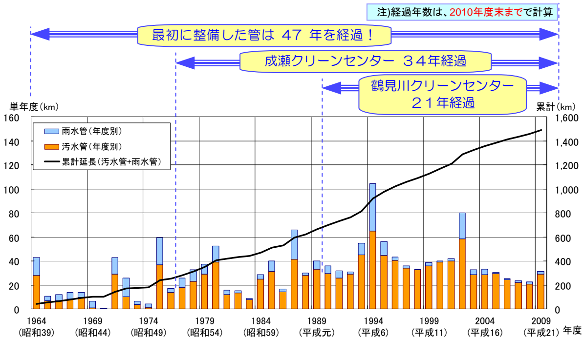
図 43 下水道管整備延長の推移と施設の経過年数
