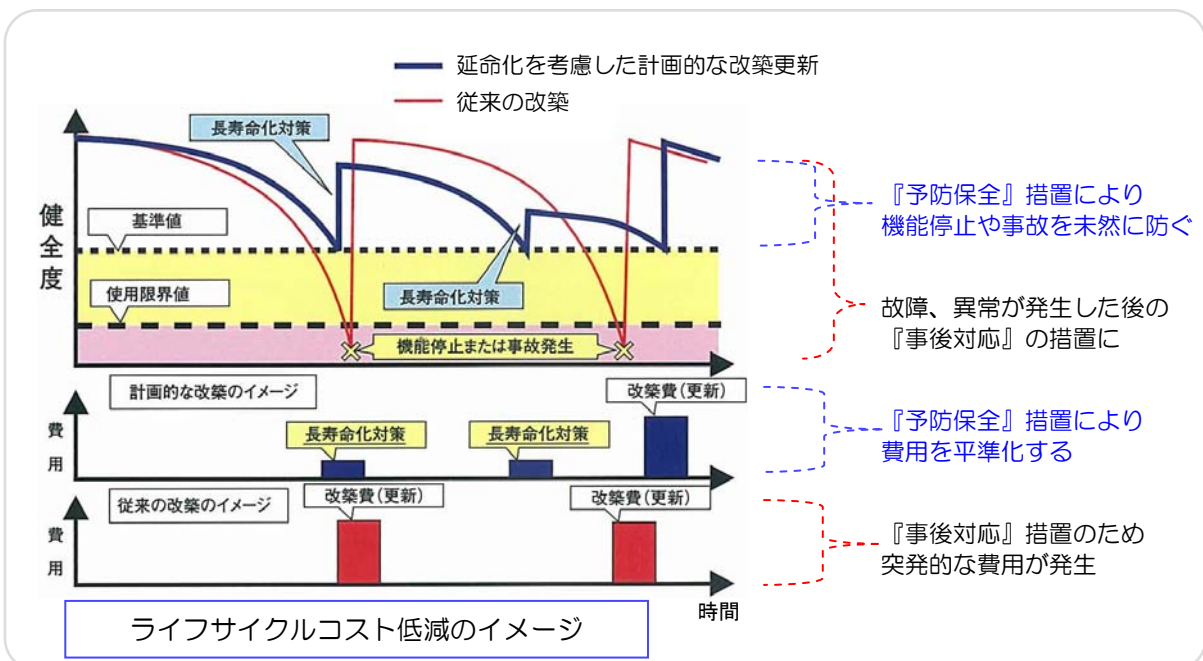
図 45 下水道施設の延命化（長寿命化）を考慮した計画的な改築更新（ストックマネジメント）
