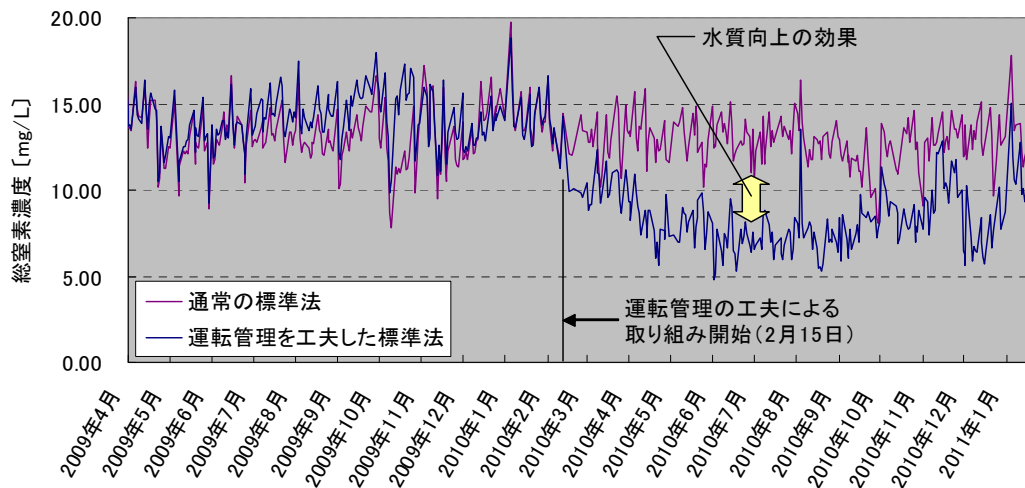
図 26 通常の標準法と運転管理を工夫した標準法との処理水質の違い (窒素での比較)
