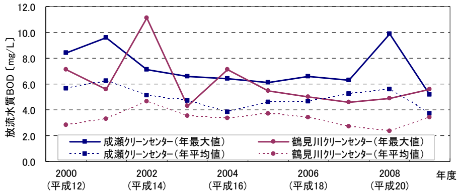
図 27 放流水質の状況
