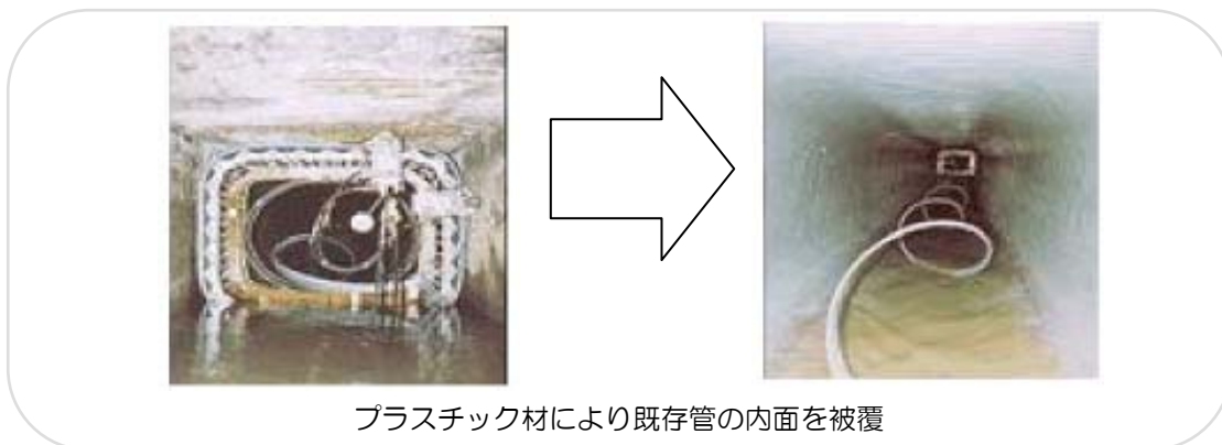
図 46 施設の延命化（更生工法の施工事例）
