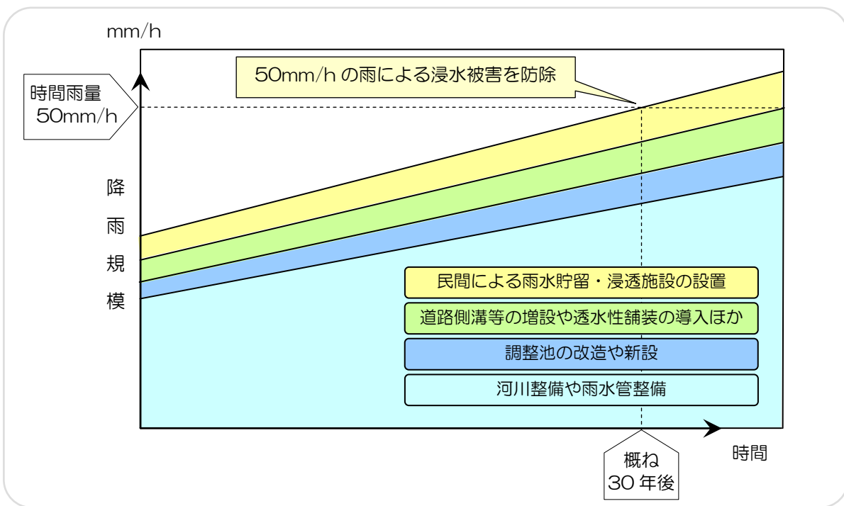
図 34 ハード対策の役割分担
