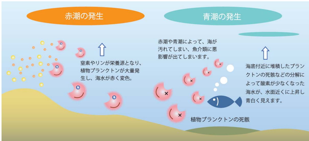
図 29 赤潮、青潮の発生メカニズム
