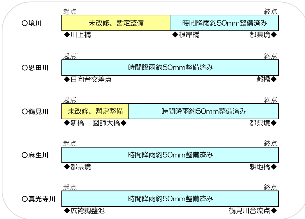
図 37 河川の整備状況 (2010 年 12 月 1 日時点)
