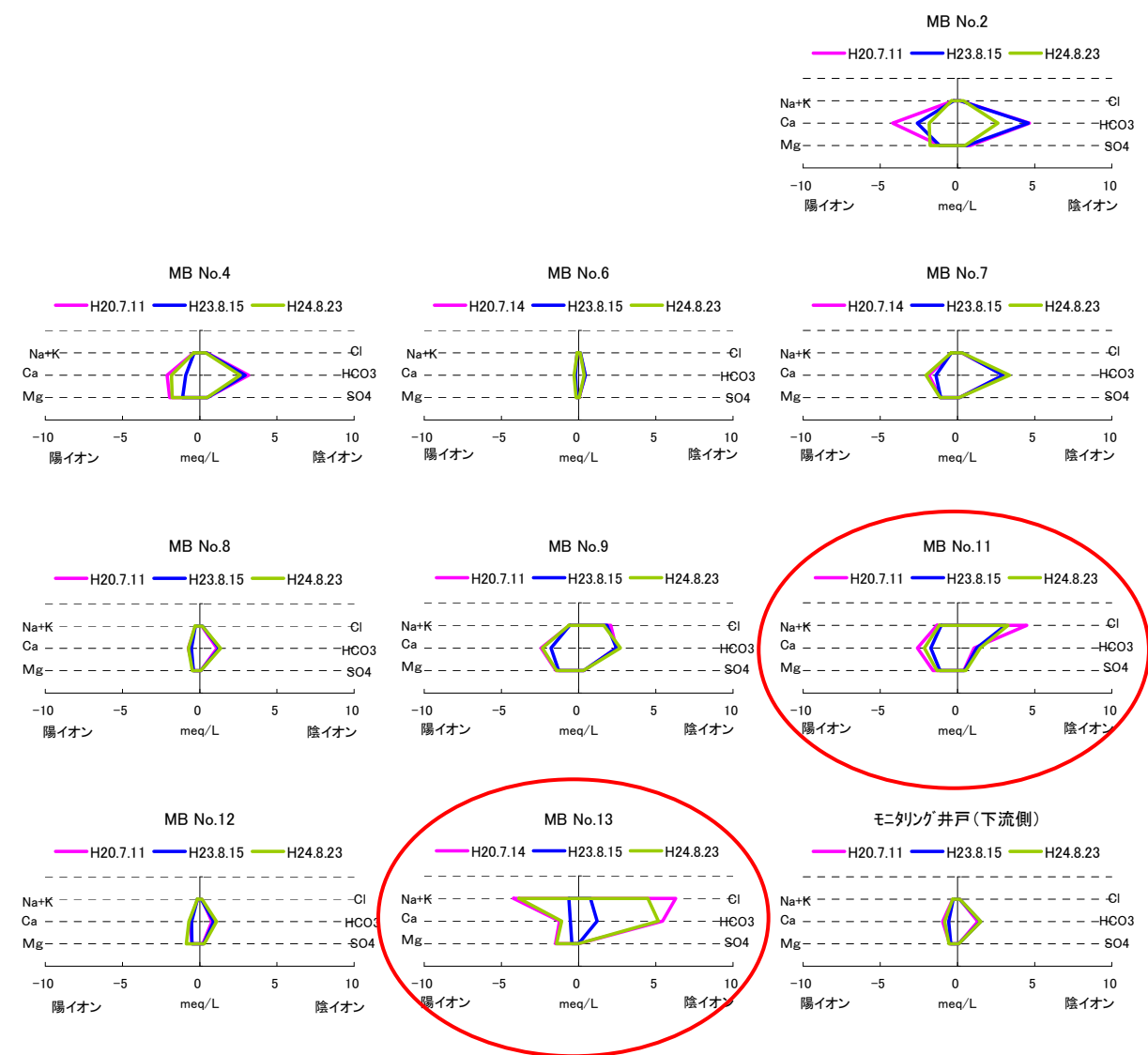
図 周辺地下水のイオンバランス
