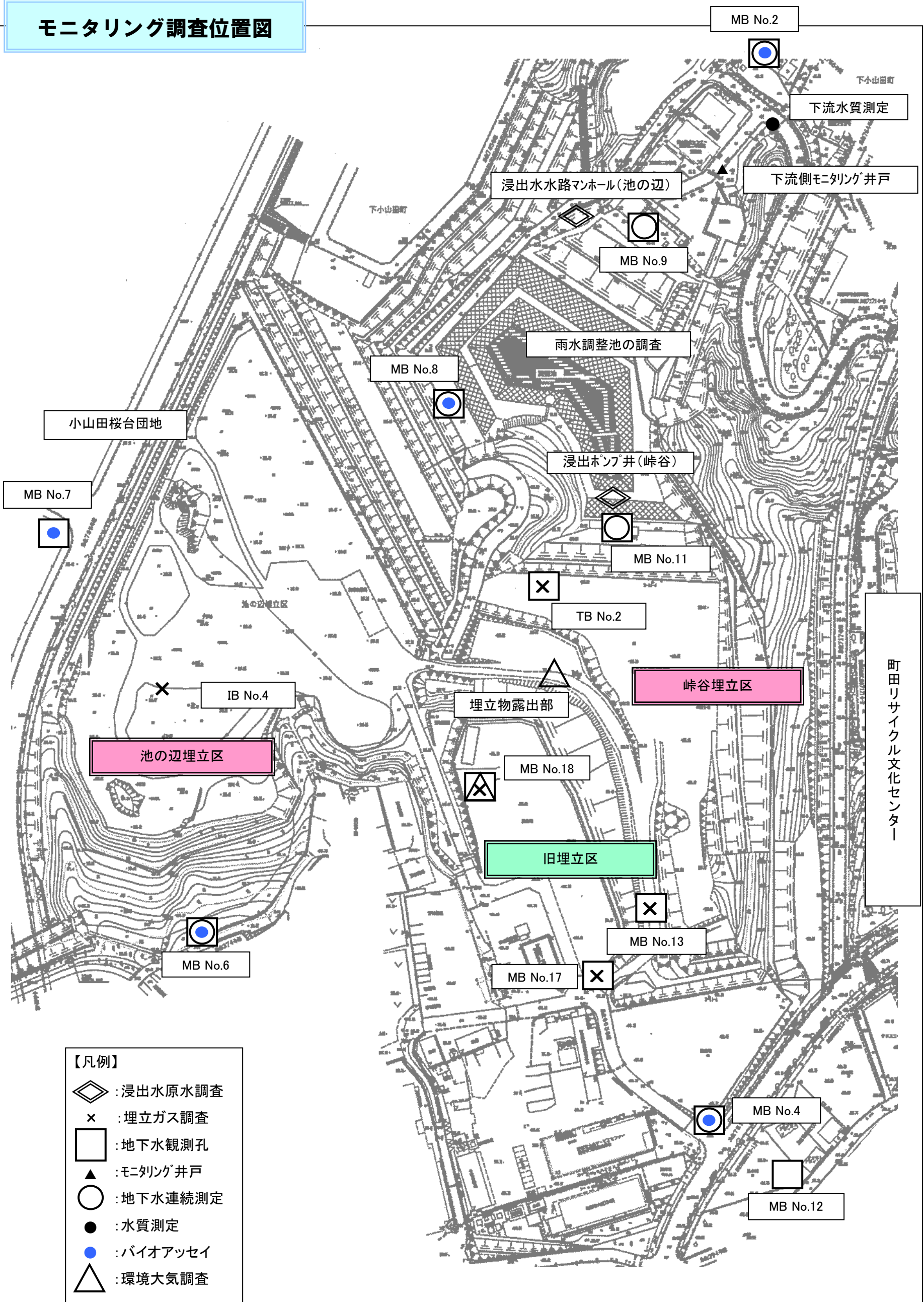
調査位置図
