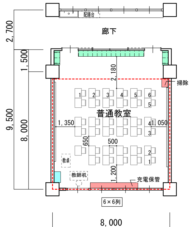
① 76m 2 (8×9.5)
