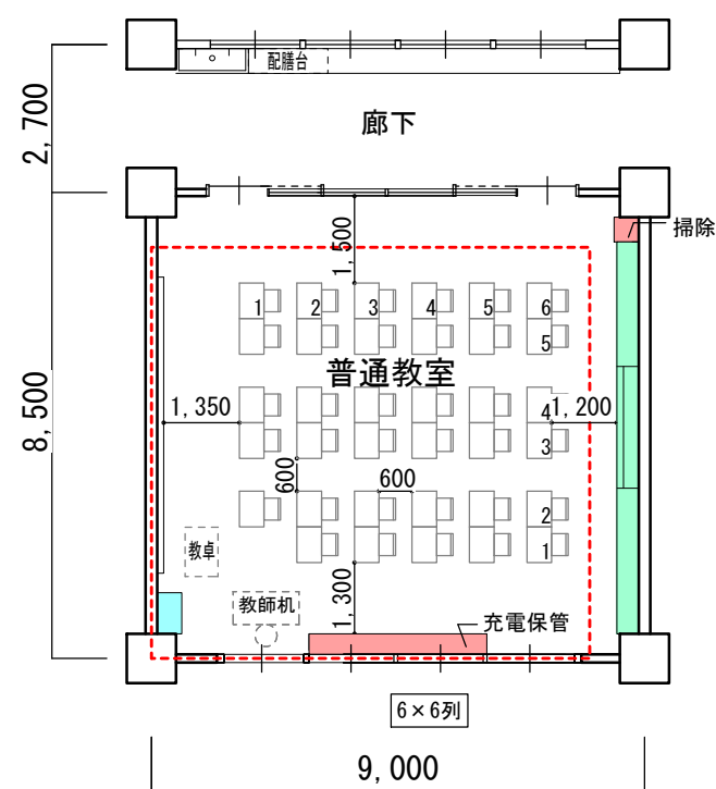
② 76m 2 (9×8.5)
