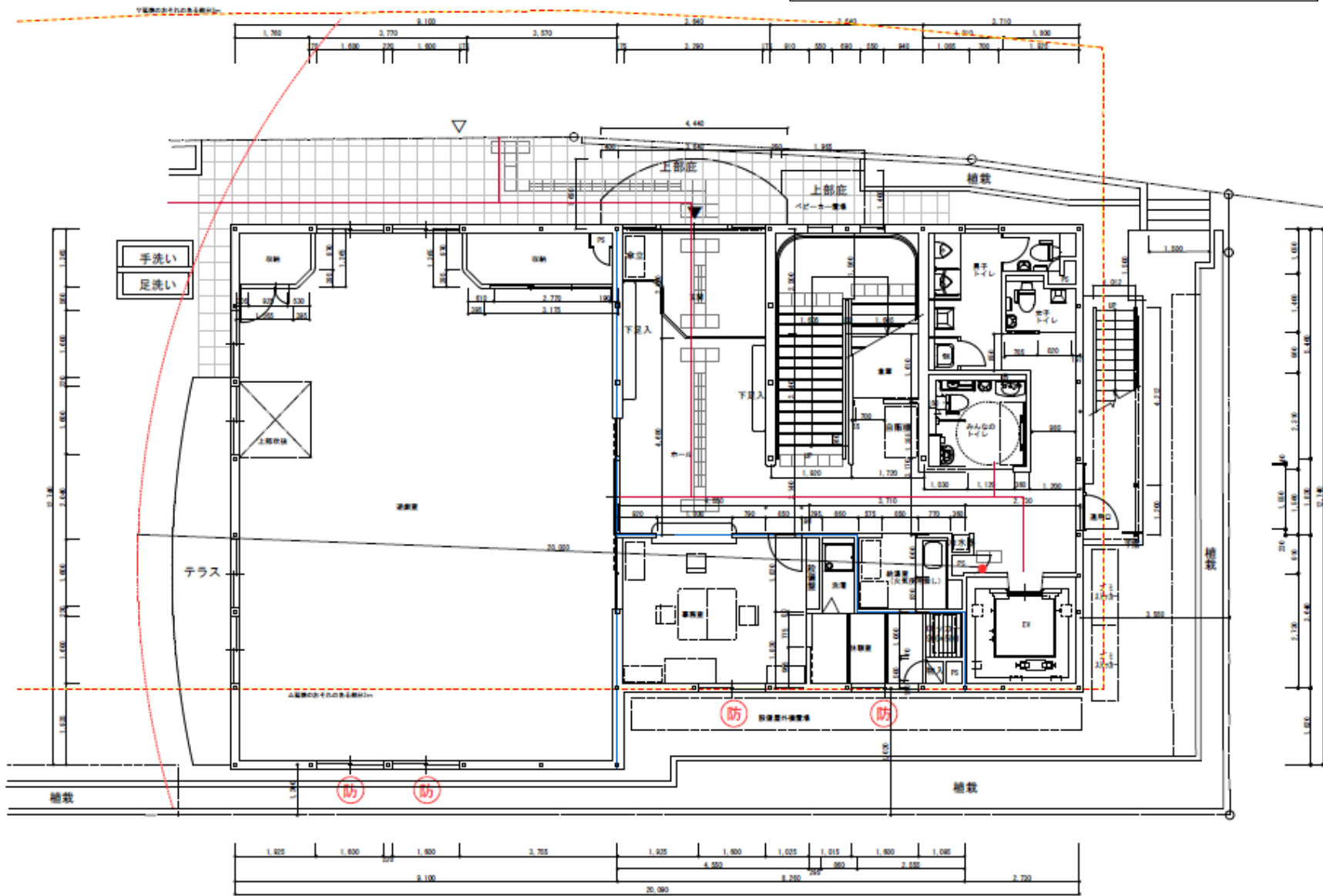
(仮称町田第三中学校区子どもクラブ 1 F 平面図案)
