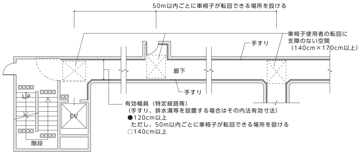
【図3.2】廊下の基本的な考え方
