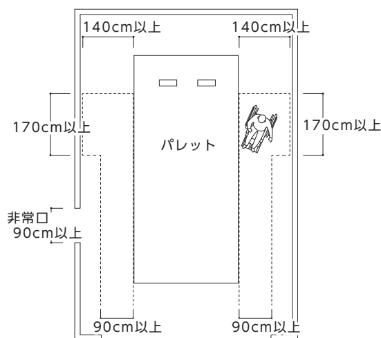
【図11.6】 機械式駐車場に車椅子使用者用駐車施設を設けた例
