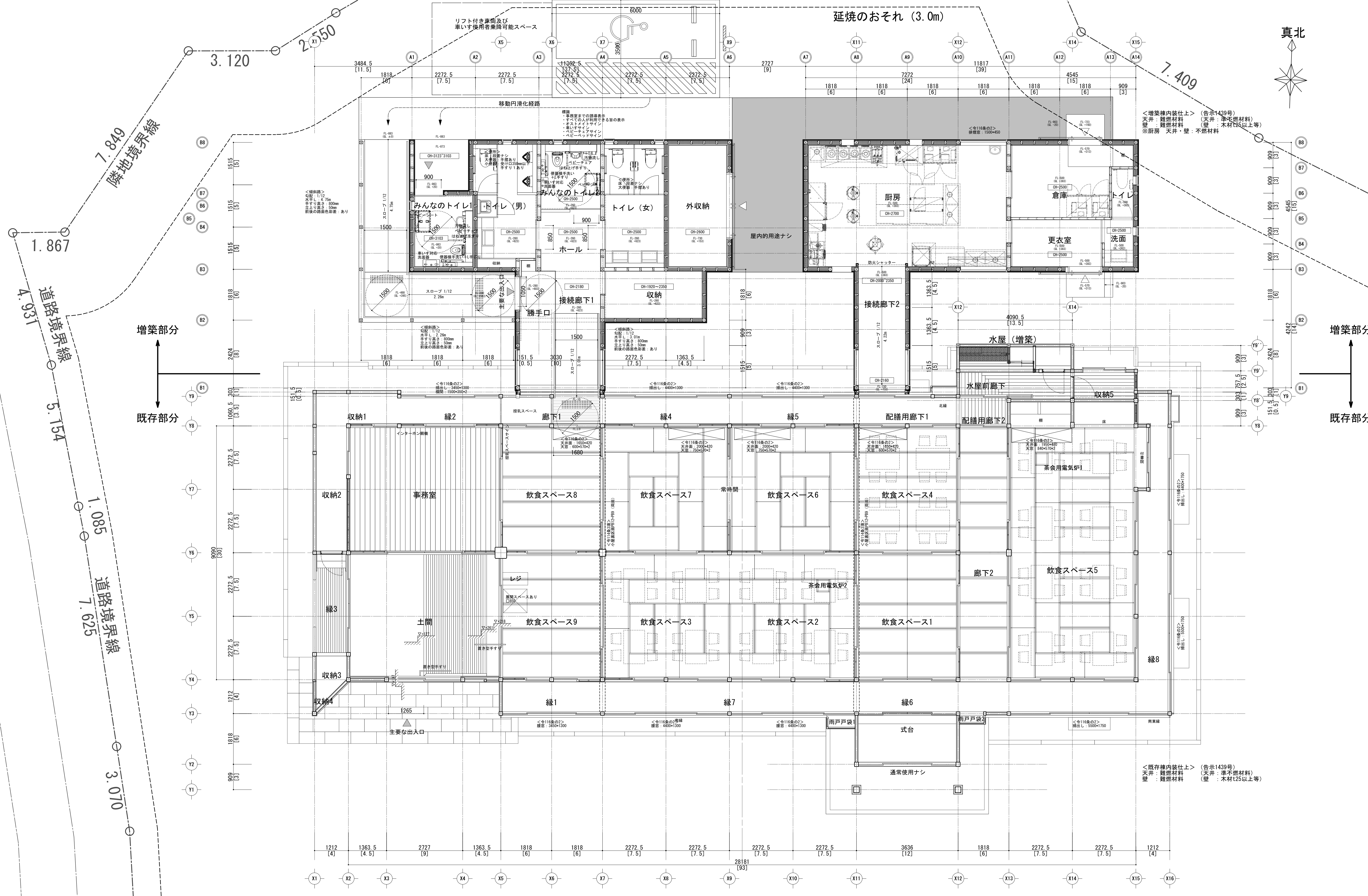
平面図
