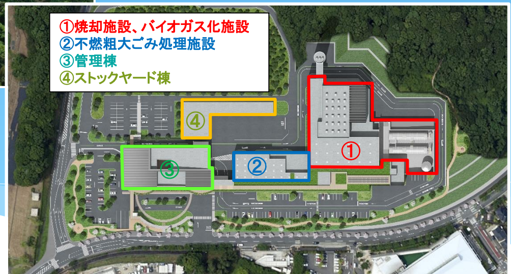
▲新しい熱回収施設等（町田リサイクル文化センター内） 配置図
