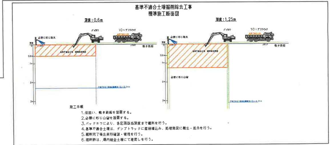
図5-2 施工方法平面・断面図
