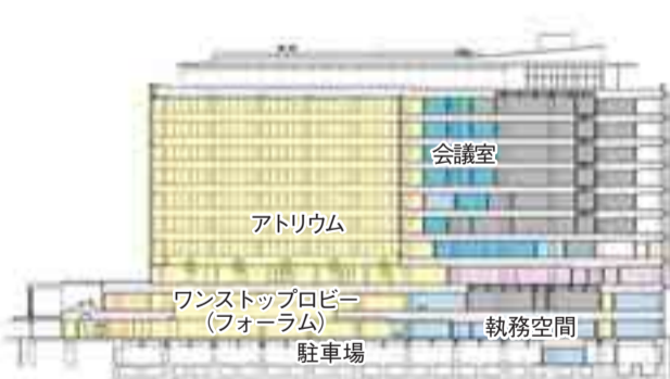
北南断面図
