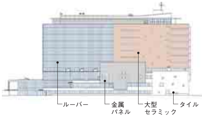
西立面図
