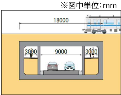
小田急線立体交差点 横断面計画図
