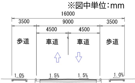
上記以外の道路部分 横断面計画図
