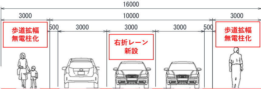
【計画断面図（標準図）】 ※図中単位：mm
