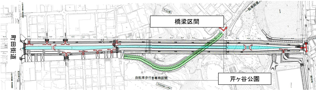
【道路平面計画図】
