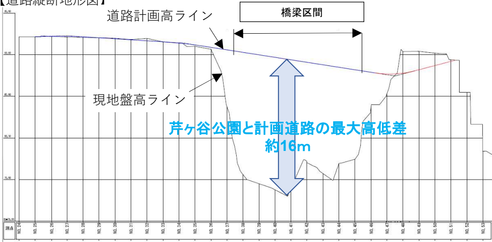
【道路縦断地形図】
