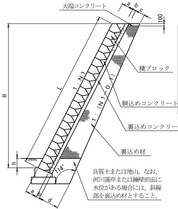
寸 法 表
