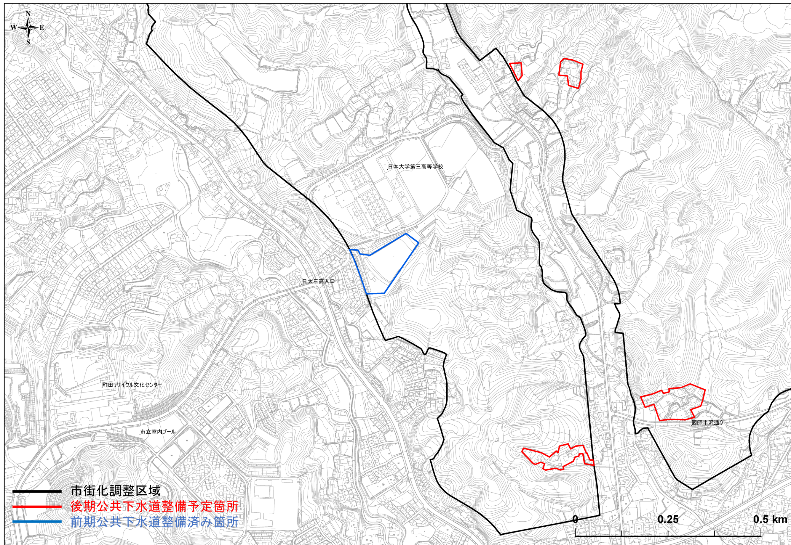
図-7 公共下水道整備計画図 (6/8)
