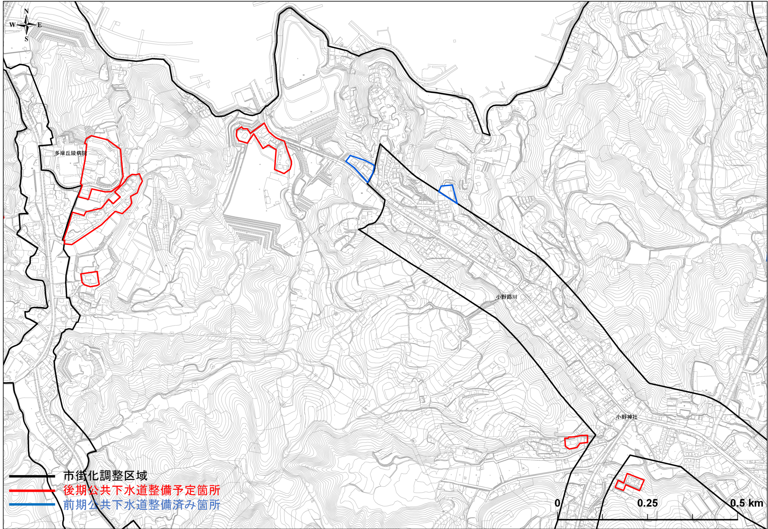
図-7 公共下水道整備計画図 (4/8)
