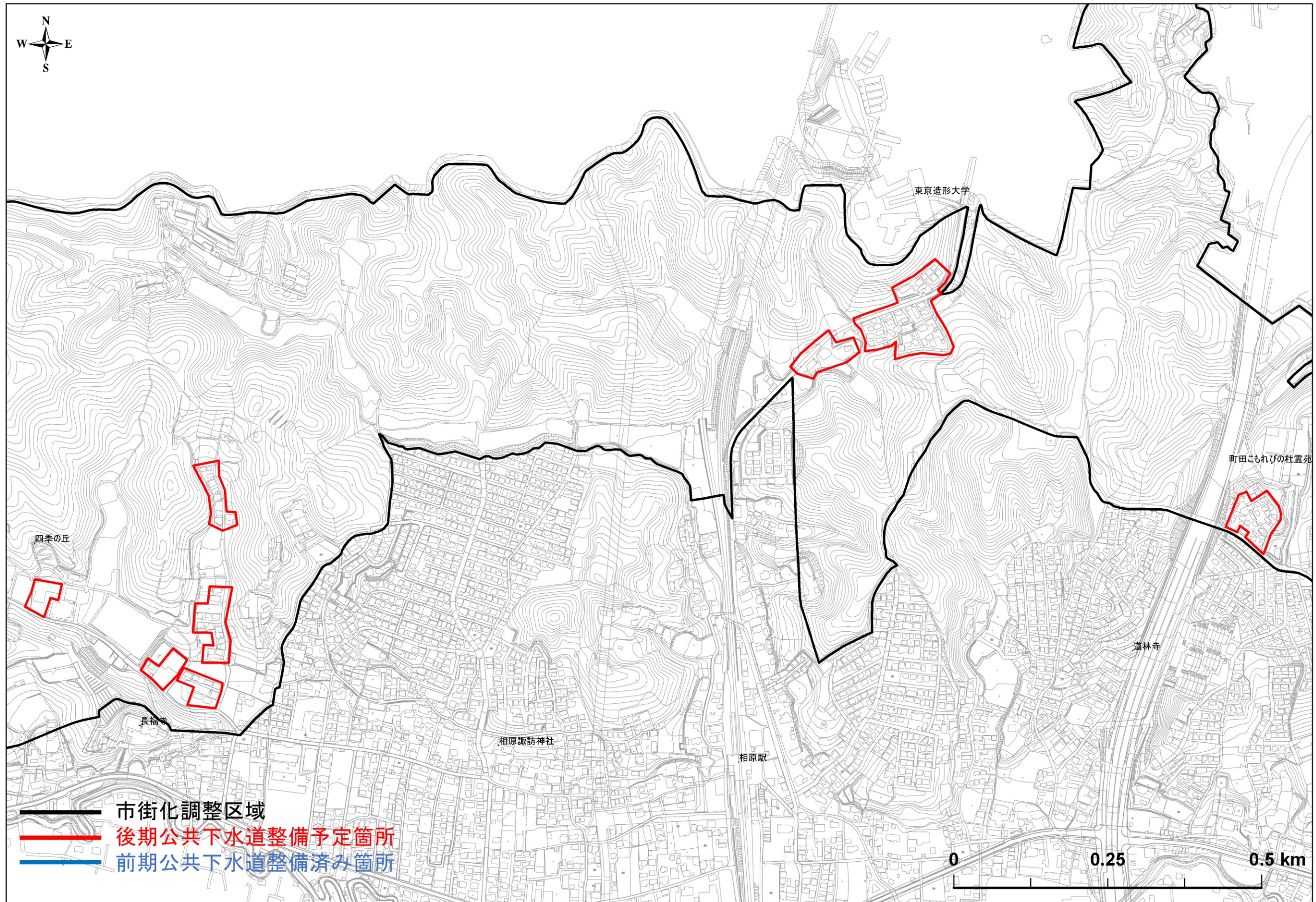
図-7 公共下水道整備計画図 (2/8)
