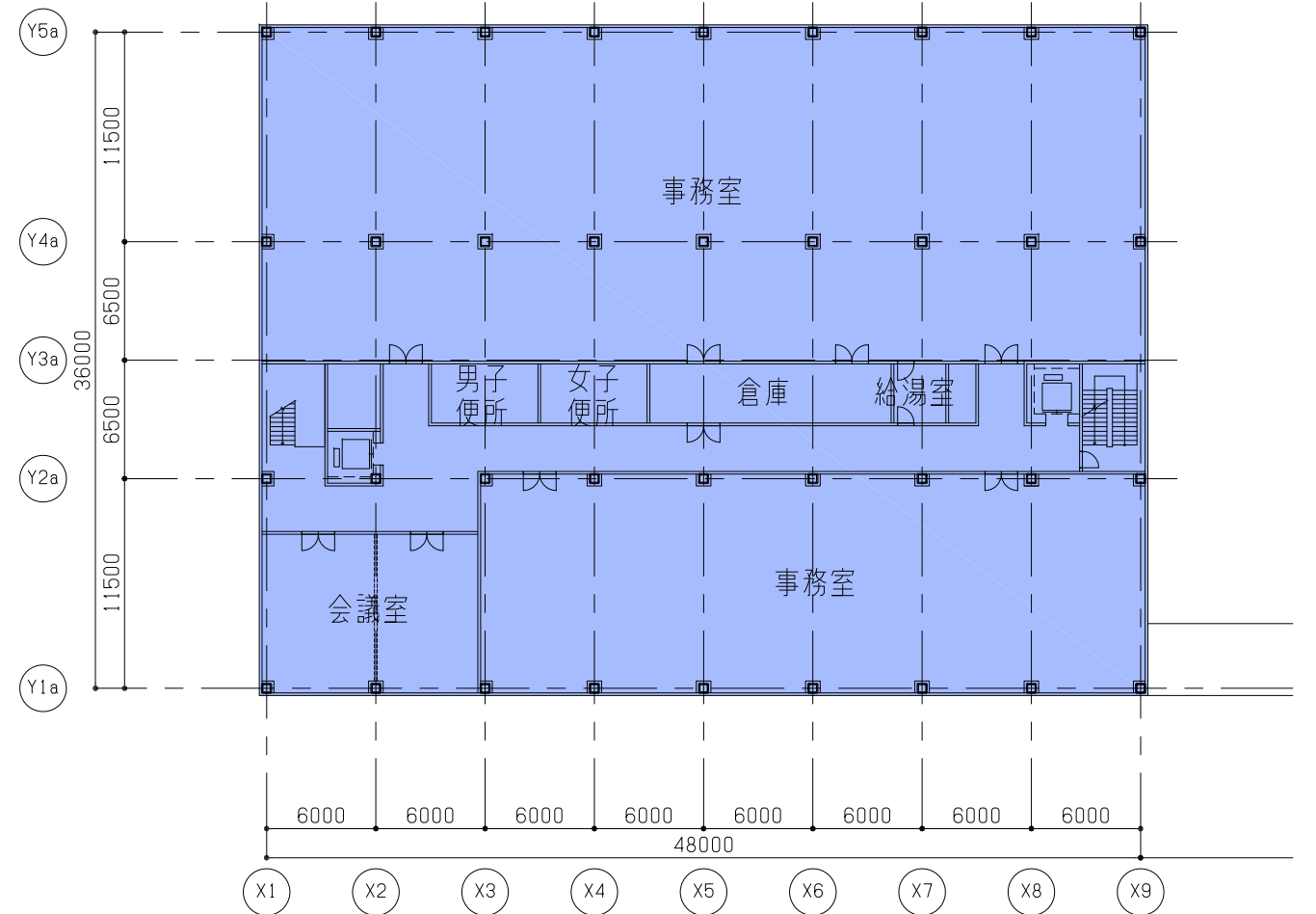
3階平面図
