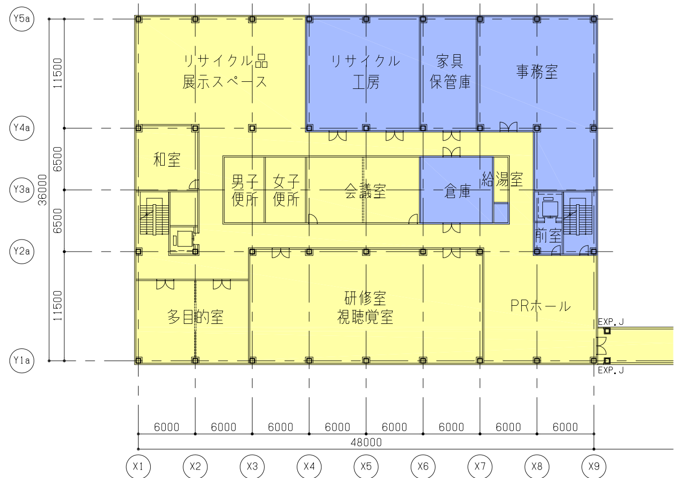
2階平面図
