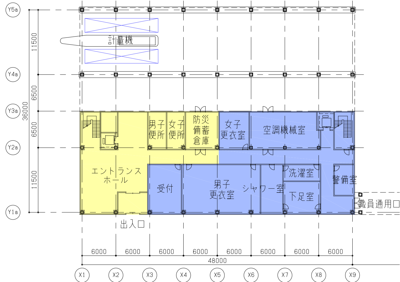
1階平面図
