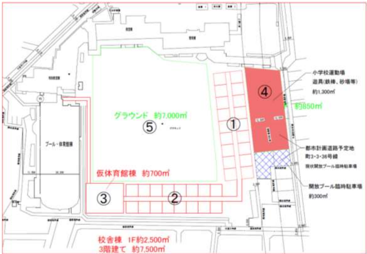
＜図 8-1＞ 仮校舎の配置案
